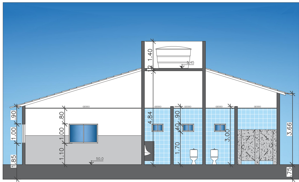
CORTE CC esc 100/10
