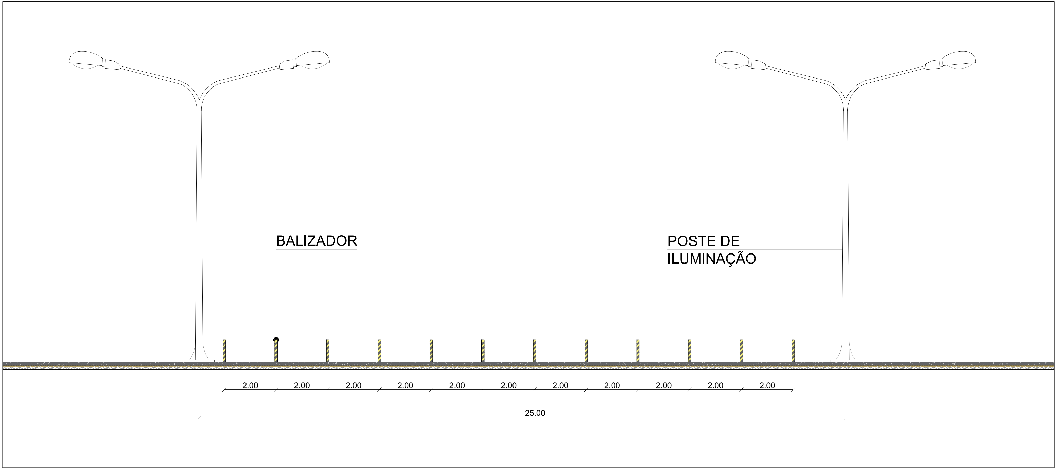
ELEVAÇÃO - TRECHO II - CALÇADÃO Escala — 1:75
