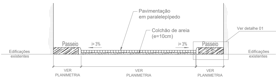
Seção Transversal tipo escala 1:100
