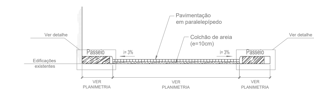
Seção Transversal tipo escala 1:100
