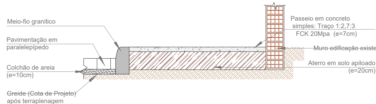
Detalhe 01 escala 1:25
